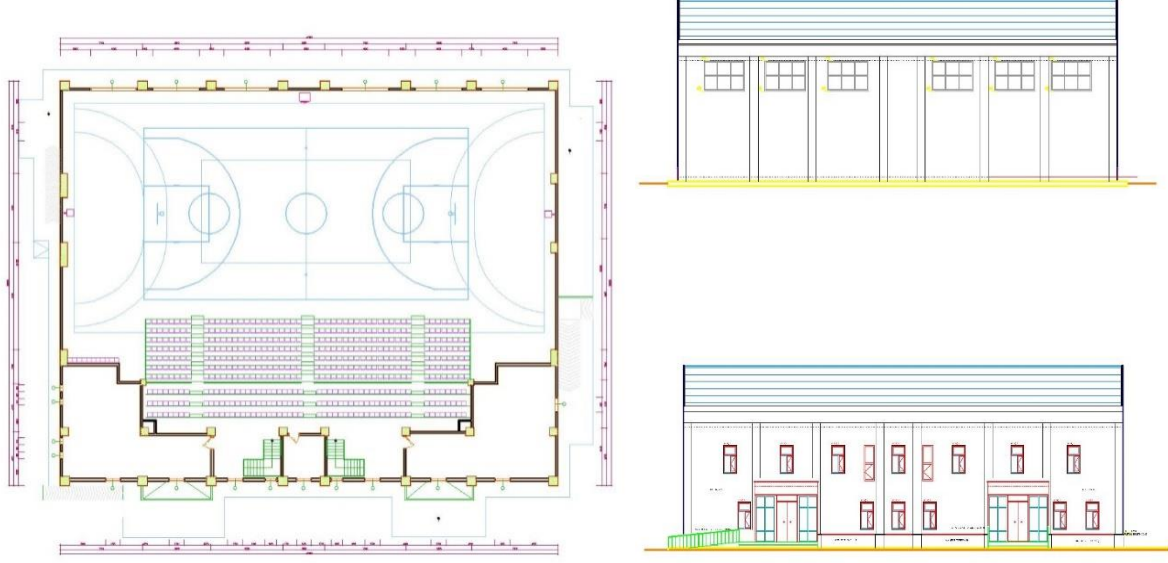
Resim 19: Ermenek 500 Kişilik Spor Salonu Mimari Görselleri
