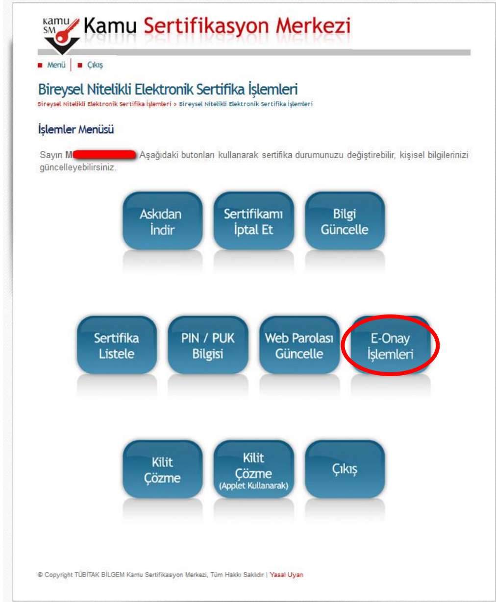
Şekil 12: İşlemler Menüsü
