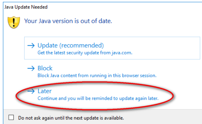
Şekil 4: Java Ekranı
