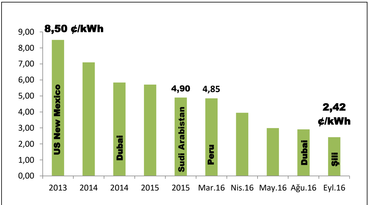
Şekil 13: 2013-2016 Dünya Alım Garantili GES İhale Fiyat Gelişimi
